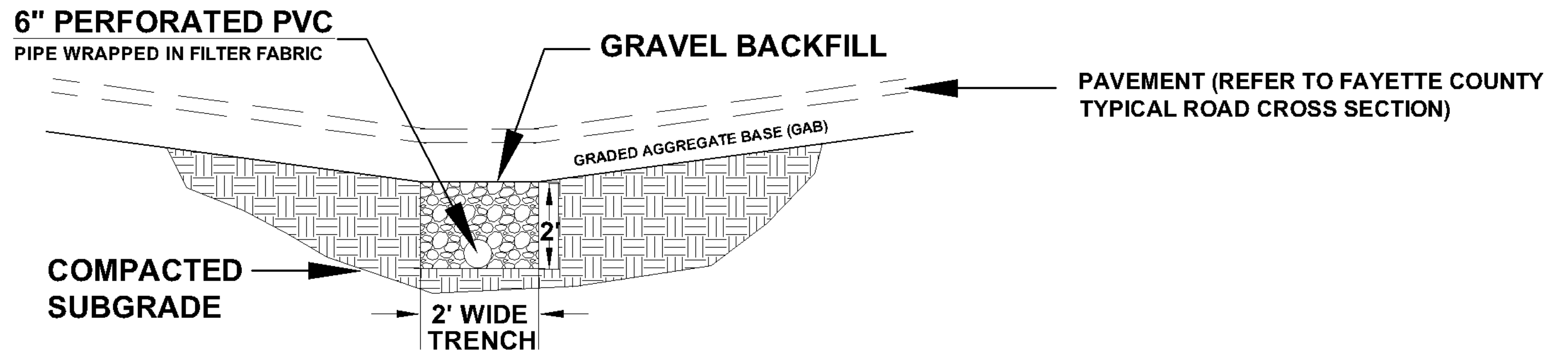
SECTION A-A'
